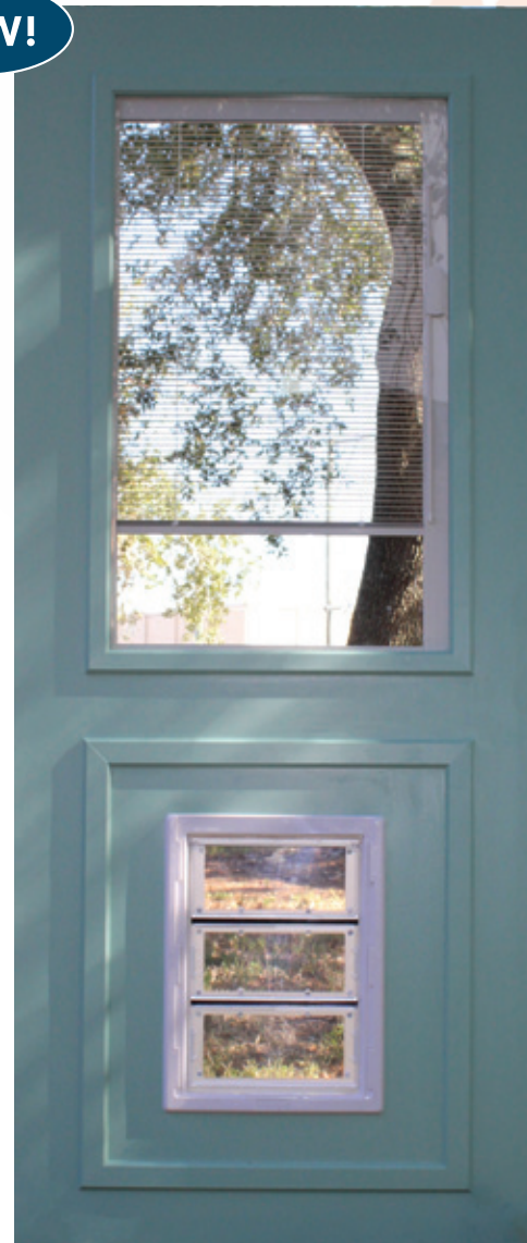
1/2 Blind Lite Over Guard Door Pet Door # 2
